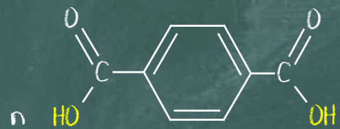
Ácido tereftálico
