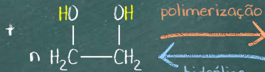
Etilenoglicol
